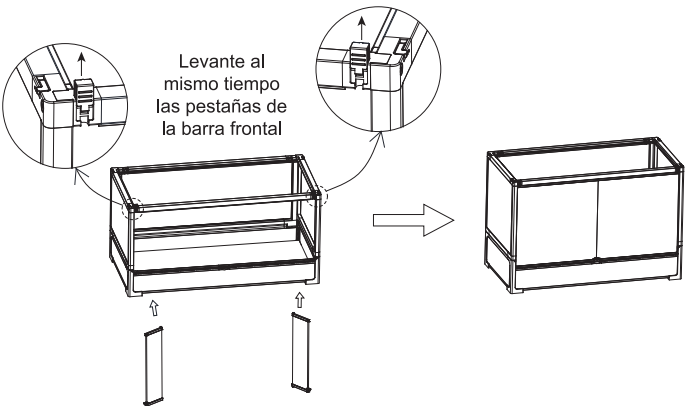
9. Monte el accesorio pasacable
