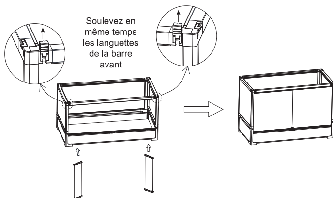
9. Montez l'accessoire passe-câble
