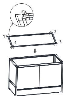
10. Ouvrez les languettes de la grille supérieure et placez-la horizontalement sur le terrarium
