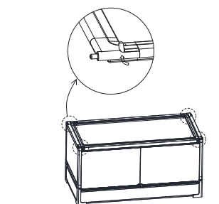
11. Fixez la grille supérieure en fermant les languettes des coins comme indiqué sur l'image
