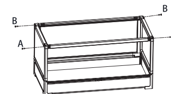
7. Utilisez les vis A pour visser et fixer les coins du panneau avant, et les vis B pour les coins du panneau arrière
