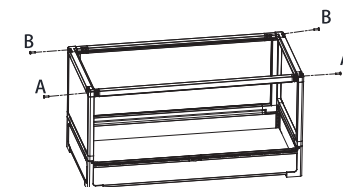
7. Utilize os parafusos A para aparafusar e fixar os cantos do painel frontal, e os parafusos B para os cantos do painel traseiro
