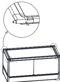
11. Asegure la malla superior cerrando las pestañas de las esquinas tal como se muestra en la imagen
